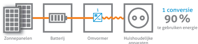
MYRESERVE: GELIJKSTROOM (DC) GEKOPPELD
